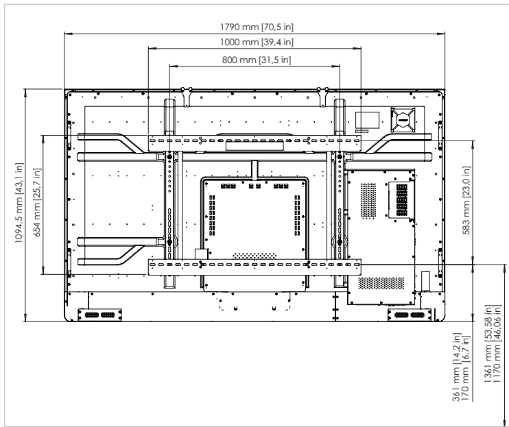
Rückansicht
