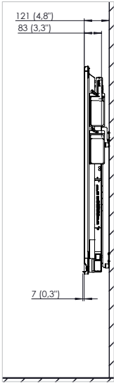
Seitenansicht
