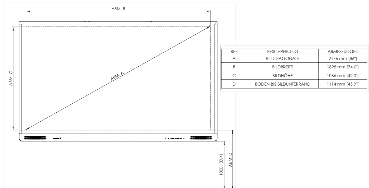
Frontansicht
