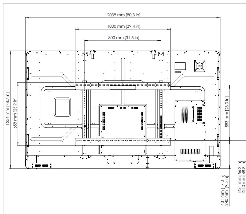
Rückansicht
