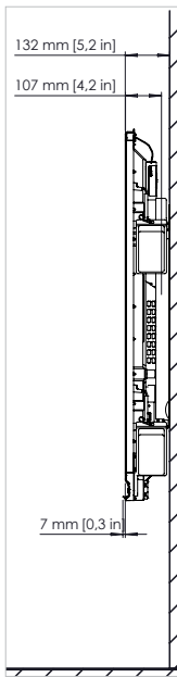
Seitenansicht
