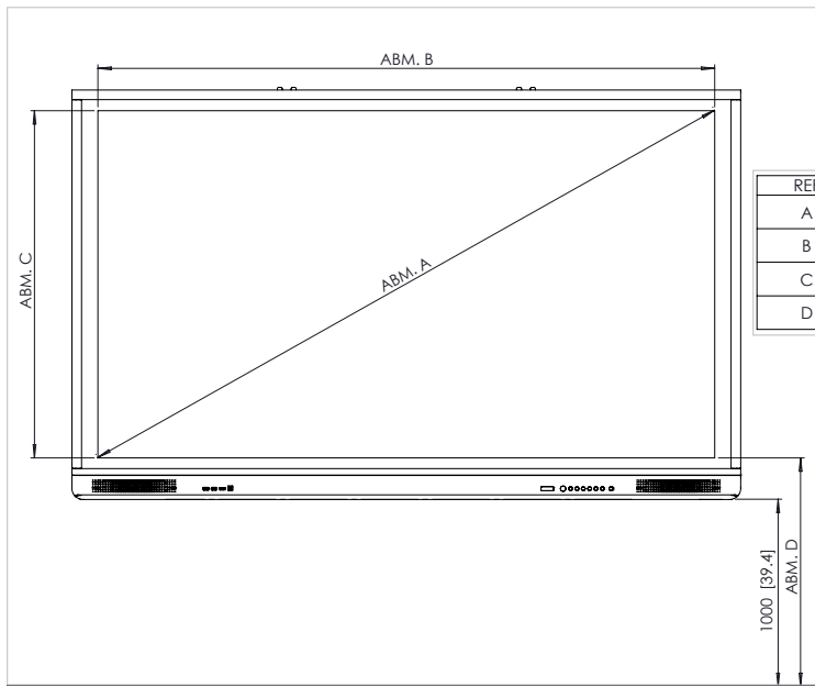
Frontansicht
