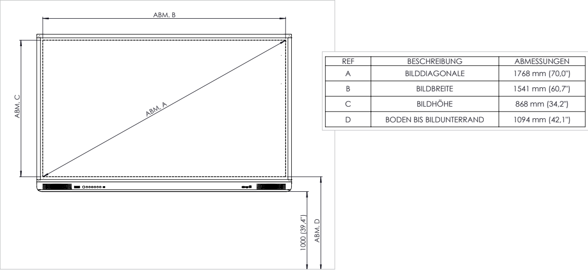
Frontansicht
