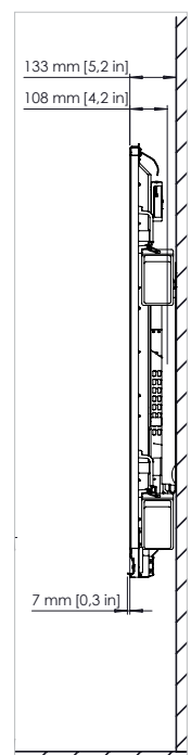
Seitenansicht
