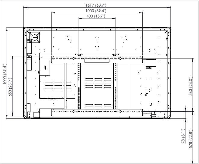
Rückansicht
