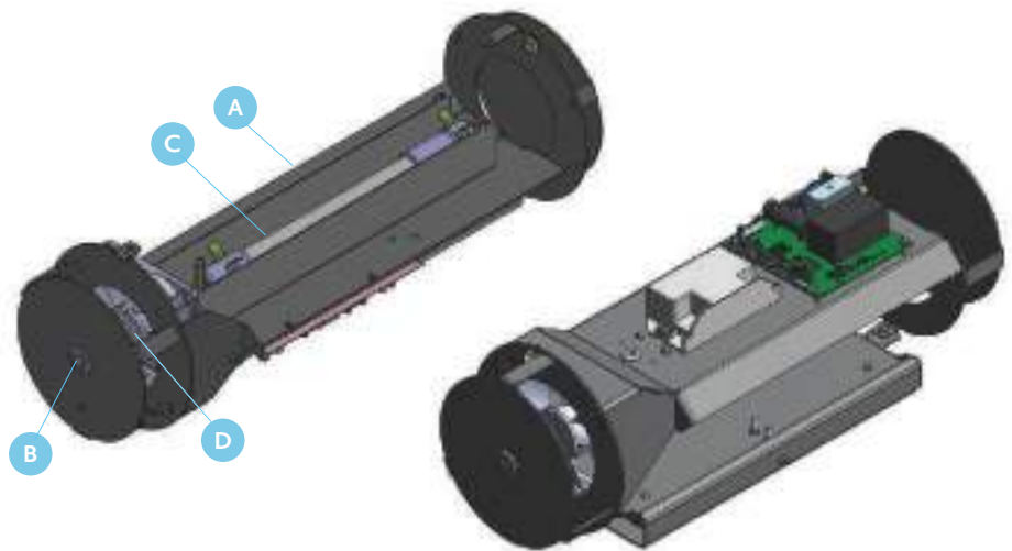
A Gehäuse · B An- / Aus-Druckschalter mit blauer Kontrollleuchte · C UV-C Spezialleuchte · D Ventilator
