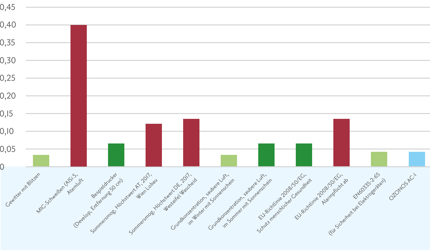
TYPISCHE OZON-KONZENTRATION IN PPM (PARTS PER MILLION)
