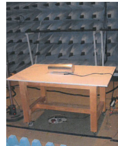
MESSUNG Spannungsschwankungen
